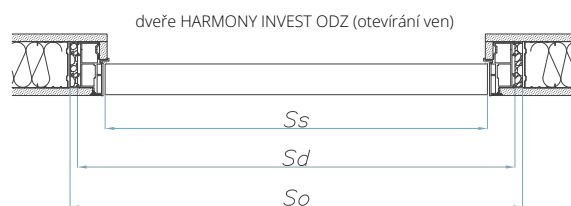
dveře HARMONY INVEST ODZ (otevírání ven)
