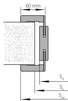
Tunel ZT s obložkami „60“
