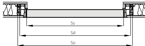
dveře ODZ (otevírání ven)
