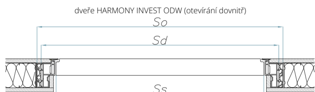
dveře HARMONY INVEST ODW (otevírání dovnitř)
