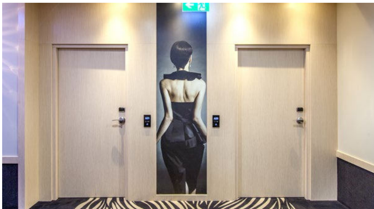
protipožární dveře FR EI30, zárubeň pevná dřevěná
