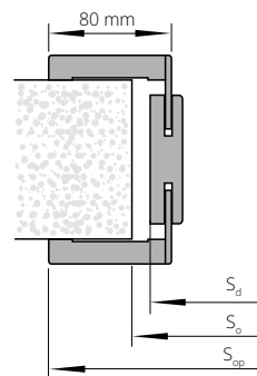
Tunel ZT s obložkami „80“
