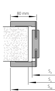
Tunel ZY s obložkami „80“
