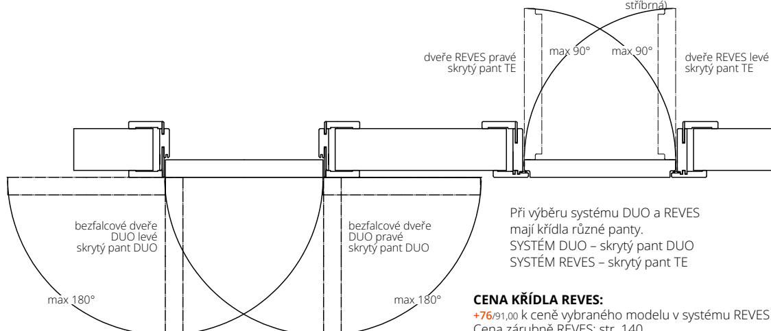
skrytý pant TE, stříbrná barva – systém REVES (kapsa pantu je černá a pohyblivá část stříbrná)
