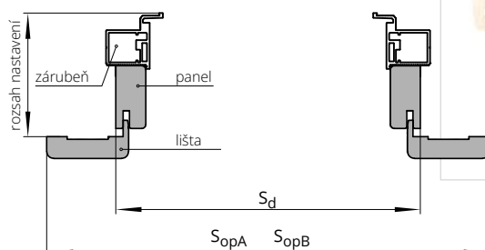
Regulační sada z MDF
